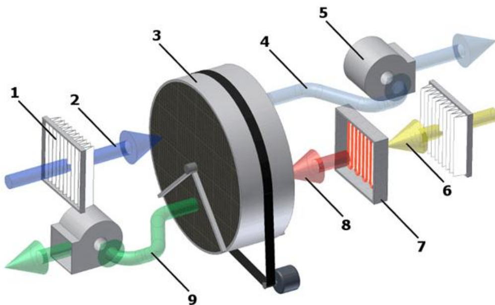
Rys. 3. Osuszacz adsorpcyjny
