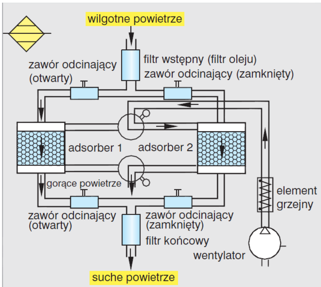
Rys. 3. Osuszacz adsorpcyjny
