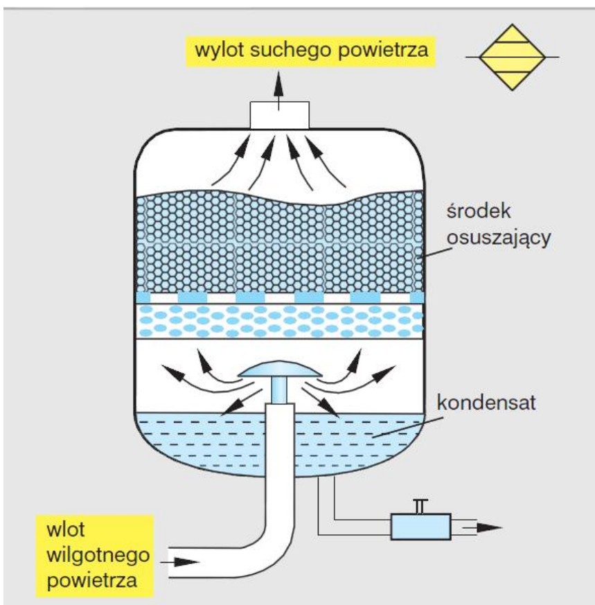
Rys. 2. Osuszacz absorpcyjny
