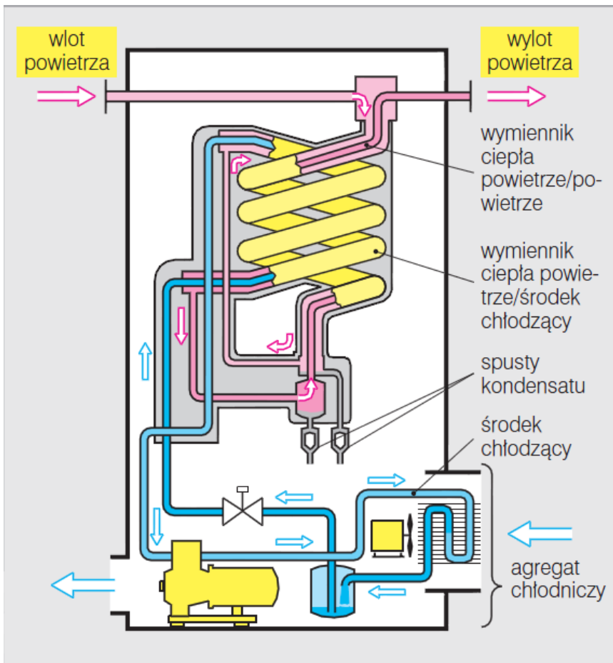
Rys. 1. Osuszacz oziębiający
